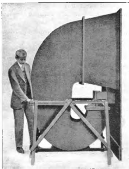
De Mondopening van dezen luidspreker heeft een afmeting van 130 bij 1.60 M.
