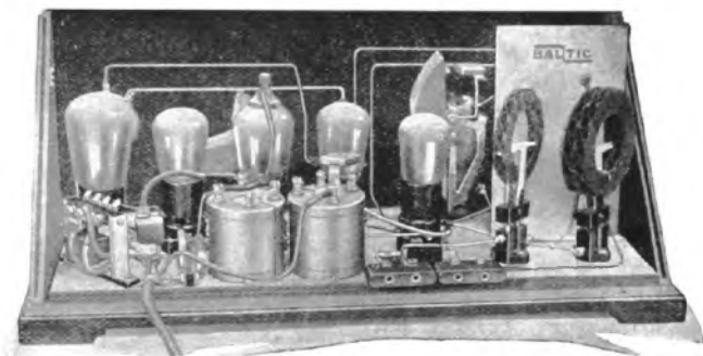
Achteraanzicht van het toestel
